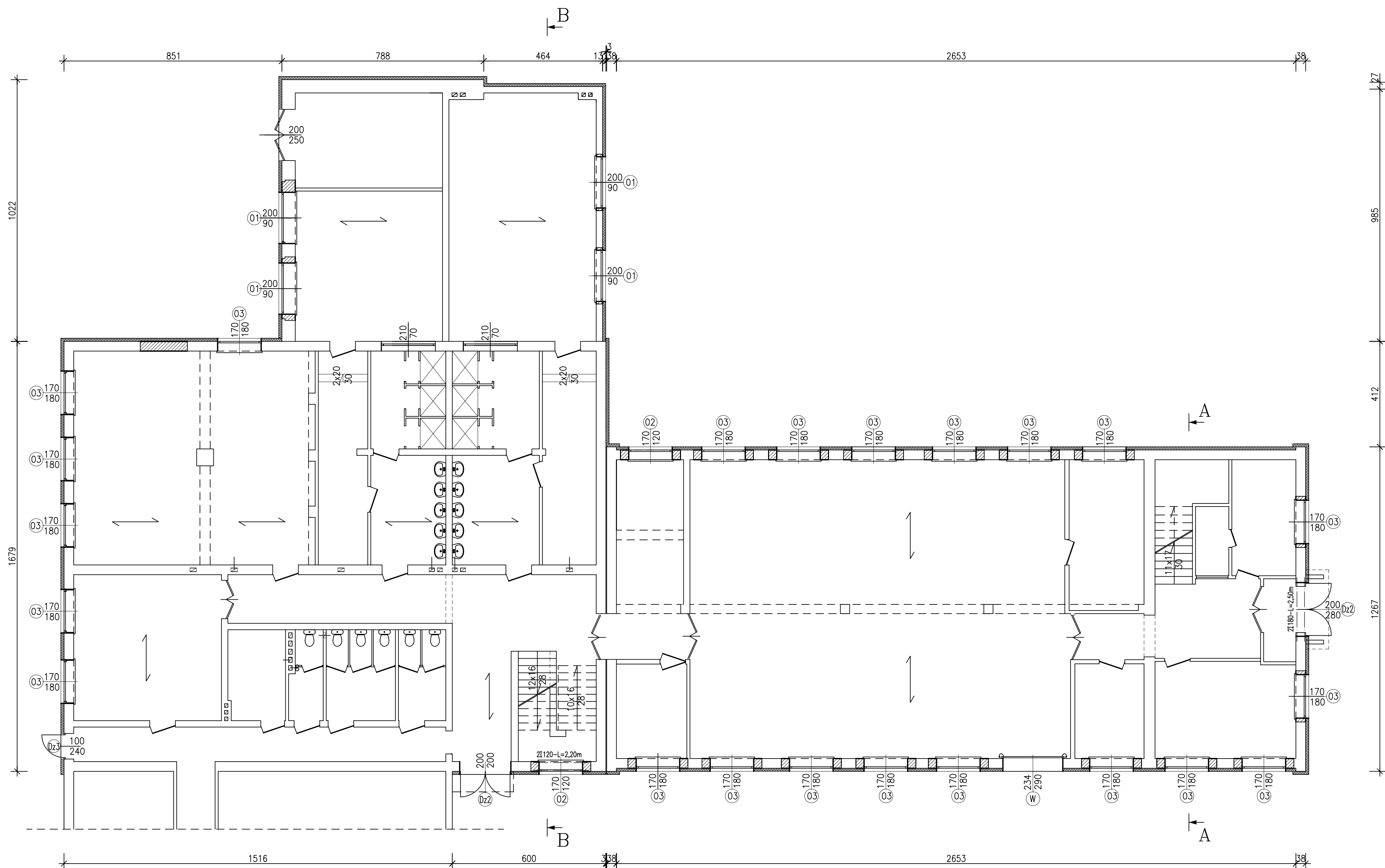
RZUT PARTERU 1:100
